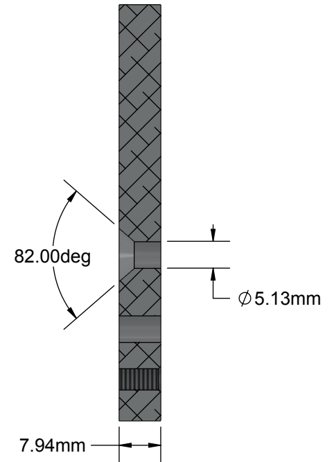
SECTION A-A
