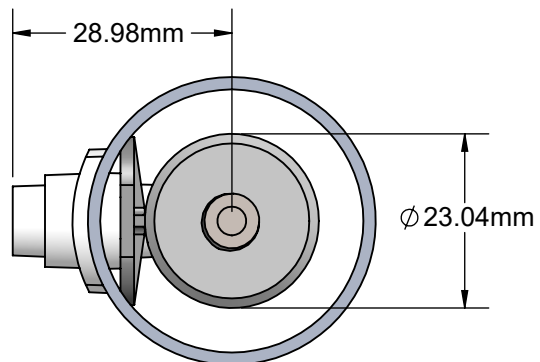
SI-111 22° FOV
