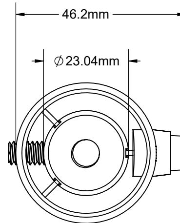
SIL-111 22° FOV
